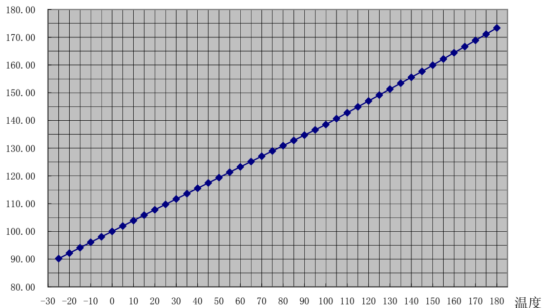
温度—阻值曲线图
