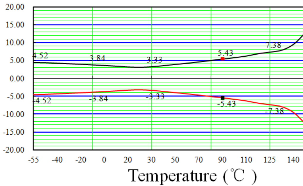
华巨电子KTY82-151测温最大偏差 °C
